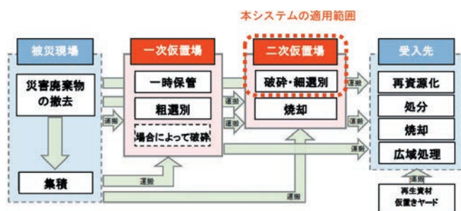
災害廃棄物の流れと本システムの適用範囲
