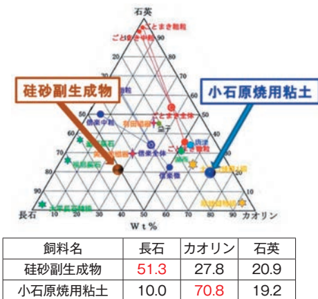
図2 硅砂副生成物の成分
