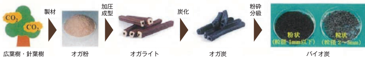
バイオ炭の製造フロー図
